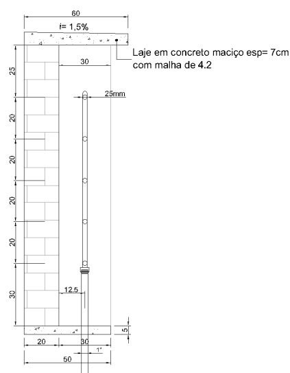
CORTE AA
