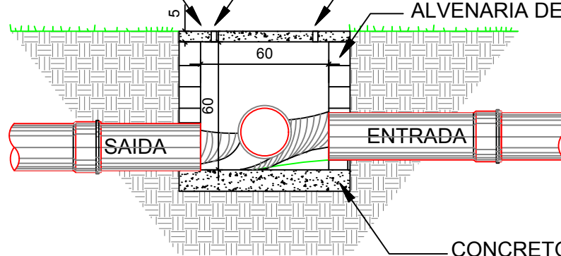
CORTE LATERAL
