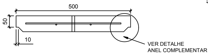
DETALHE DA TAMPA
