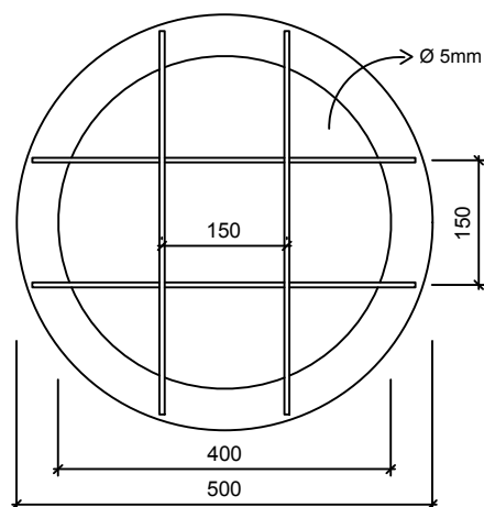
ARMAÇÃO DA TAMPA
