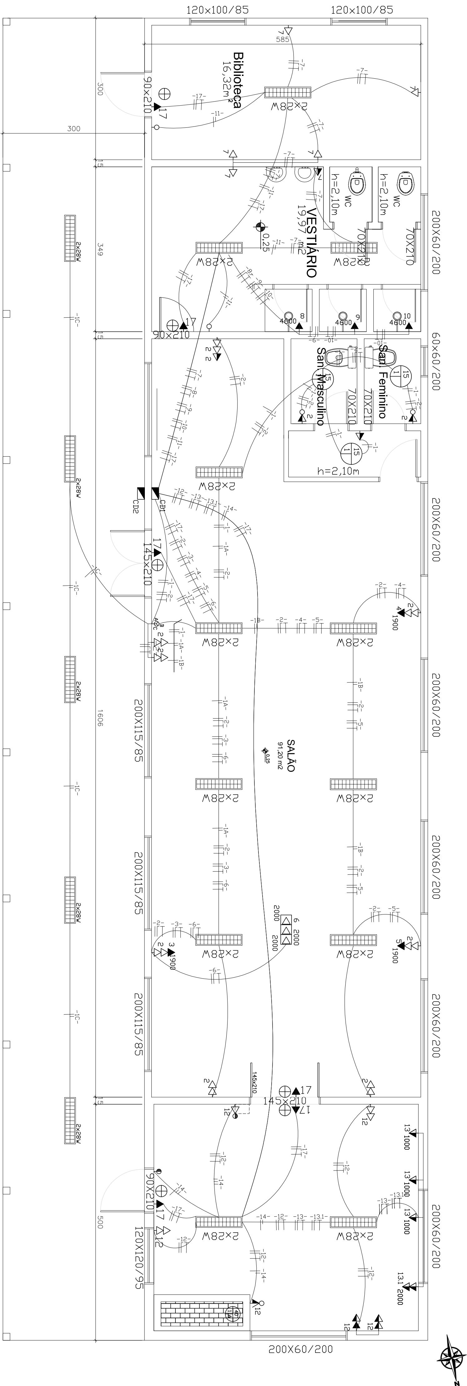
PLANTA BAIXA INSTALAÇÕES ELÉTRICAS
