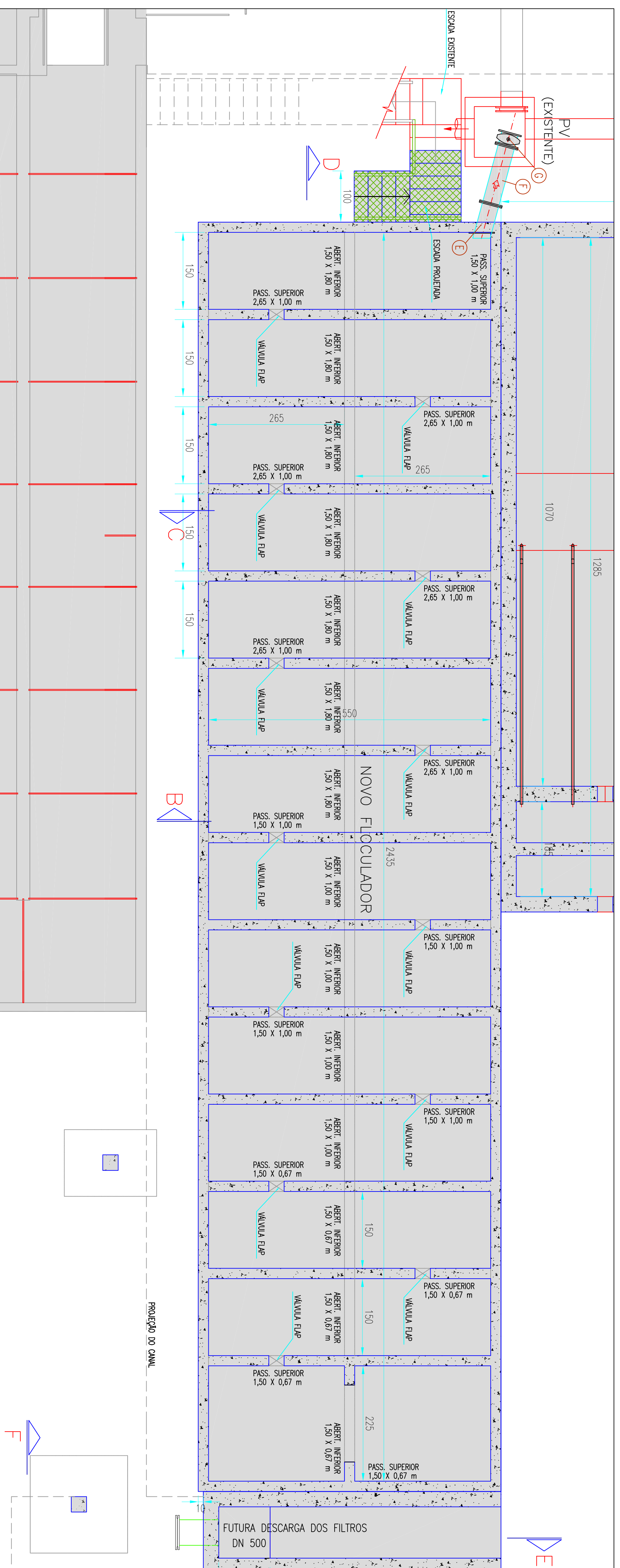
PLANTA NIVEL INFERIOR ESCALA 1:50
