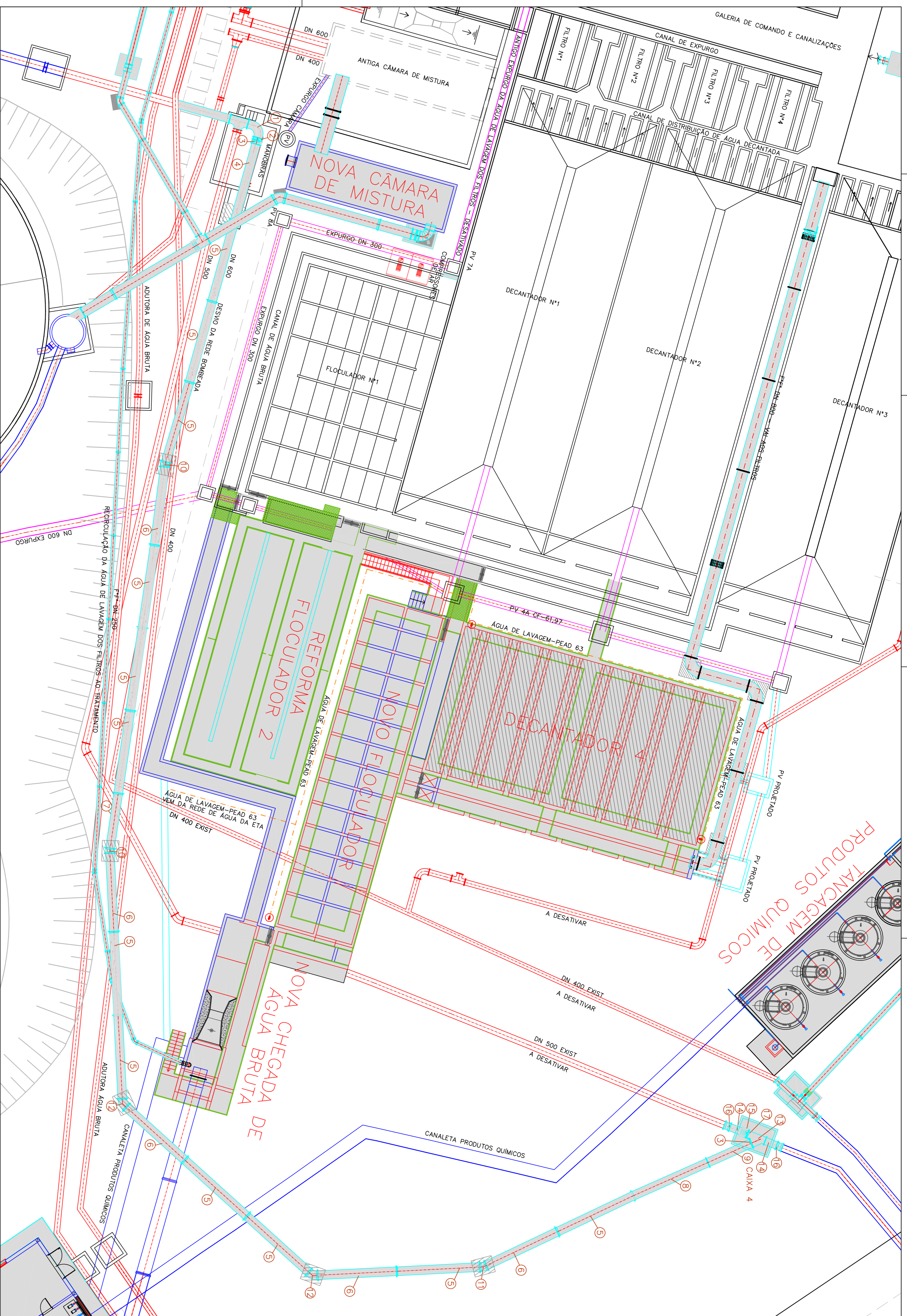
PLANTA BAIXA ESCALA 1:200
